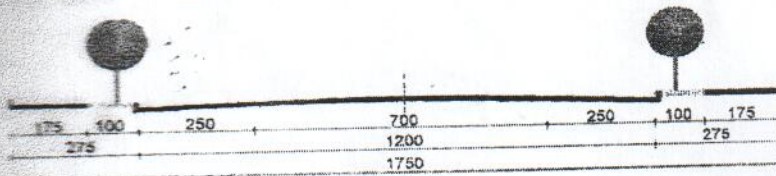
VIA DE CONTORNO E INTERIORES
